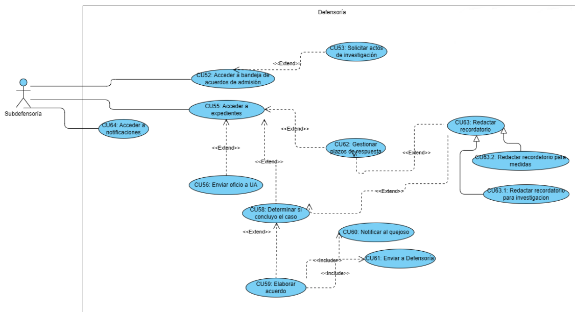
Figura 4: Diagrama de Casos de Uso del Microservicio Subdefensoría
