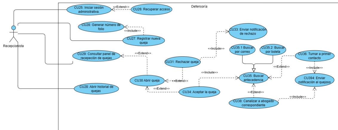
Figura 2: Diagrama de Casos de Uso del Microservicio Recepcionista
