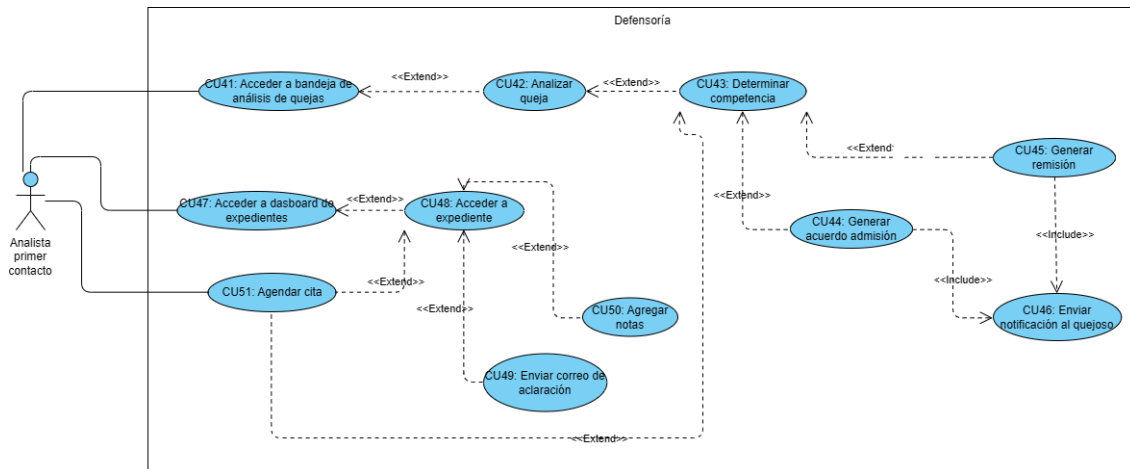
Figura 3: Diagrama de Casos de Uso del Microservicio Analista de Primer Contacto
