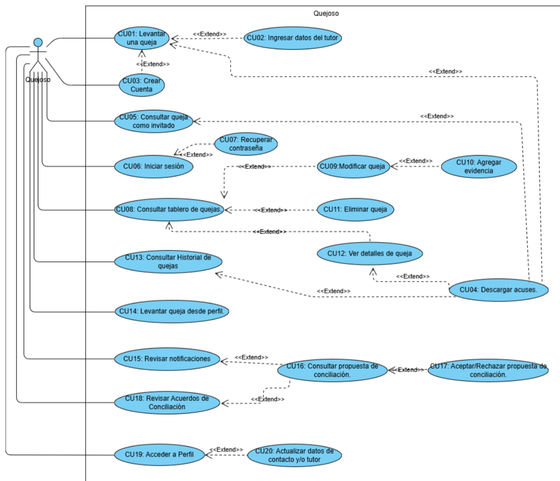
Figura 1: Diagrama de Casos de Uso del Microservicio Quejoso
