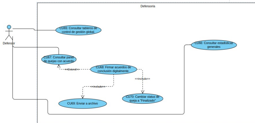
Figura 5: Diagrama de Casos de Uso del Microservicio Defensoría
